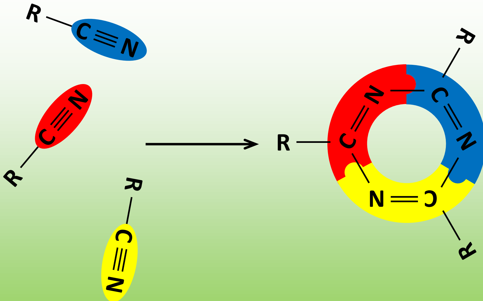
cyclootrimer
