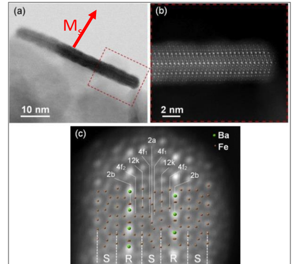
Posnetek magnetne nanoploščice z vrstičnim presevnim mikroskopom z atomsko ločljivostjo: D. Makovec, IJS (vir, Makovec in drugi, Acta Mater. 2019)
