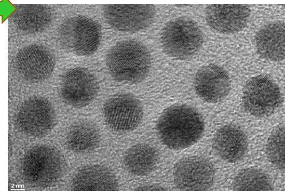
posnetek nanodelcev zlata s presevnim elektronskim mikroskopom
