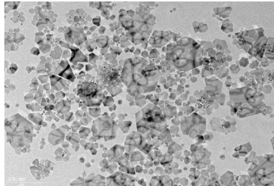
Posnetek s presevnim elektronskim mikroskopom (D. Lisjak)
