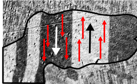
Magnetne domene zrna magnetne keramike, posnetek s Kerr-ovim mikroskopom (Zureks Wikimedia Commons)
