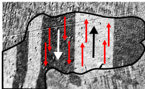
Magnetne domene zrnju magnetne keramike, posnetek s Kerr-ovim mikroskopom (Zureks Wikimedia Commons)
