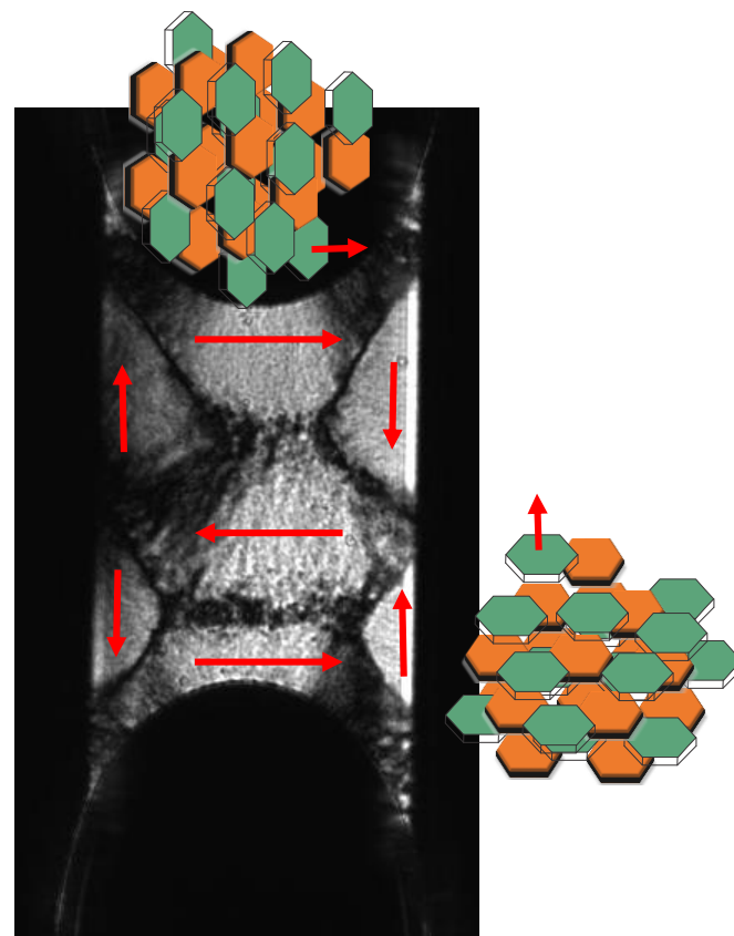
Magnetne domene v tekočem magnetu, posnetek z optičnim mikroskopom: N. Sebastian
