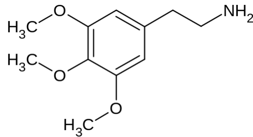
Meskalin
