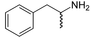
Amfetamin
