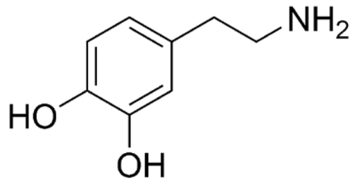
Dopamin
